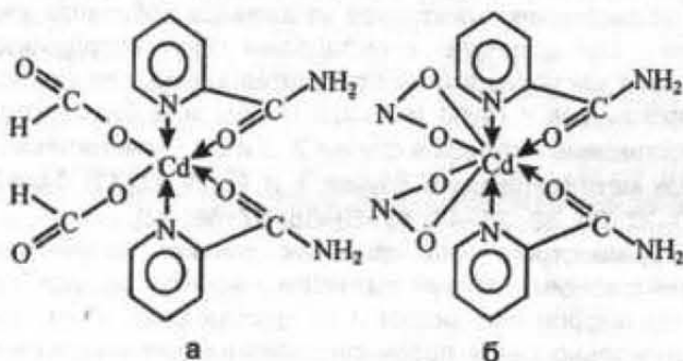
Рис. 3. Строение комплексов: а – \text{Cd}(\text{HCOO})_2(\text{ПА})_2 ; б – [\text{Cd}(\text{NO}_2)_2(\text{ПА})_2]
