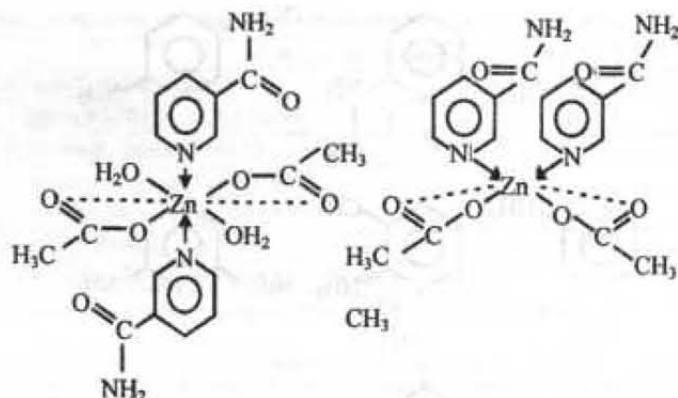
Рис. 4. Строение комплекса: [\text{Zn}(\text{CH}_3\text{COO})_2(\text{НА})_2(\text{H}_2\text{O})_2]_2 - ([\text{Zn}(\text{CH}_3\text{COO})_2(\text{НА})_2(\text{H}_2\text{O})_2])_2
