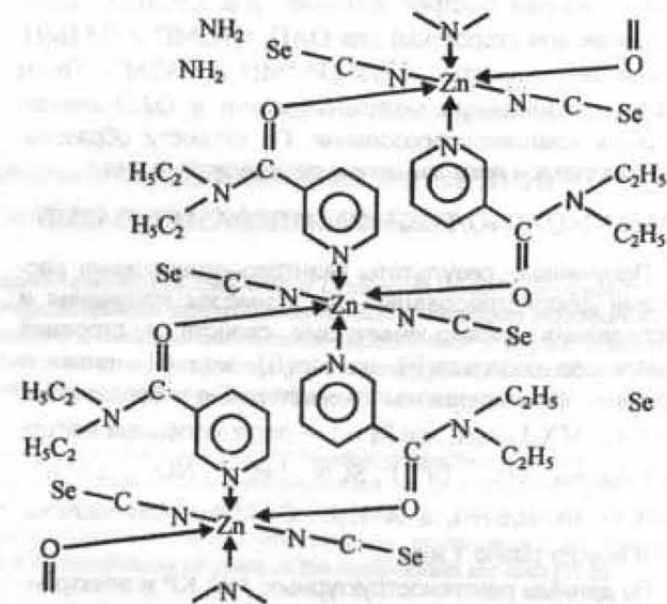
Рис. 5. Строение комплекса [\text{Zn}(\text{NCSe})_2(\text{ДЭНА})_2]
