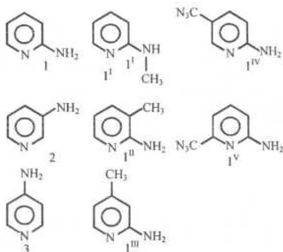
Рис. 1. 1-3 – орто-, мета-, парааминопиридины (О-, М-, ПАП); 1'-1'' – орто-амино(п)метилпиридины (ОА(п)МП – n = 2, 3, 4, 5, 6)
